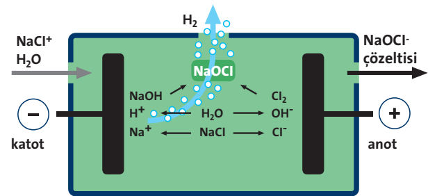
Elektrolitik hücre içerisinde sodyumhipoklorit çözeltisi üretimi
